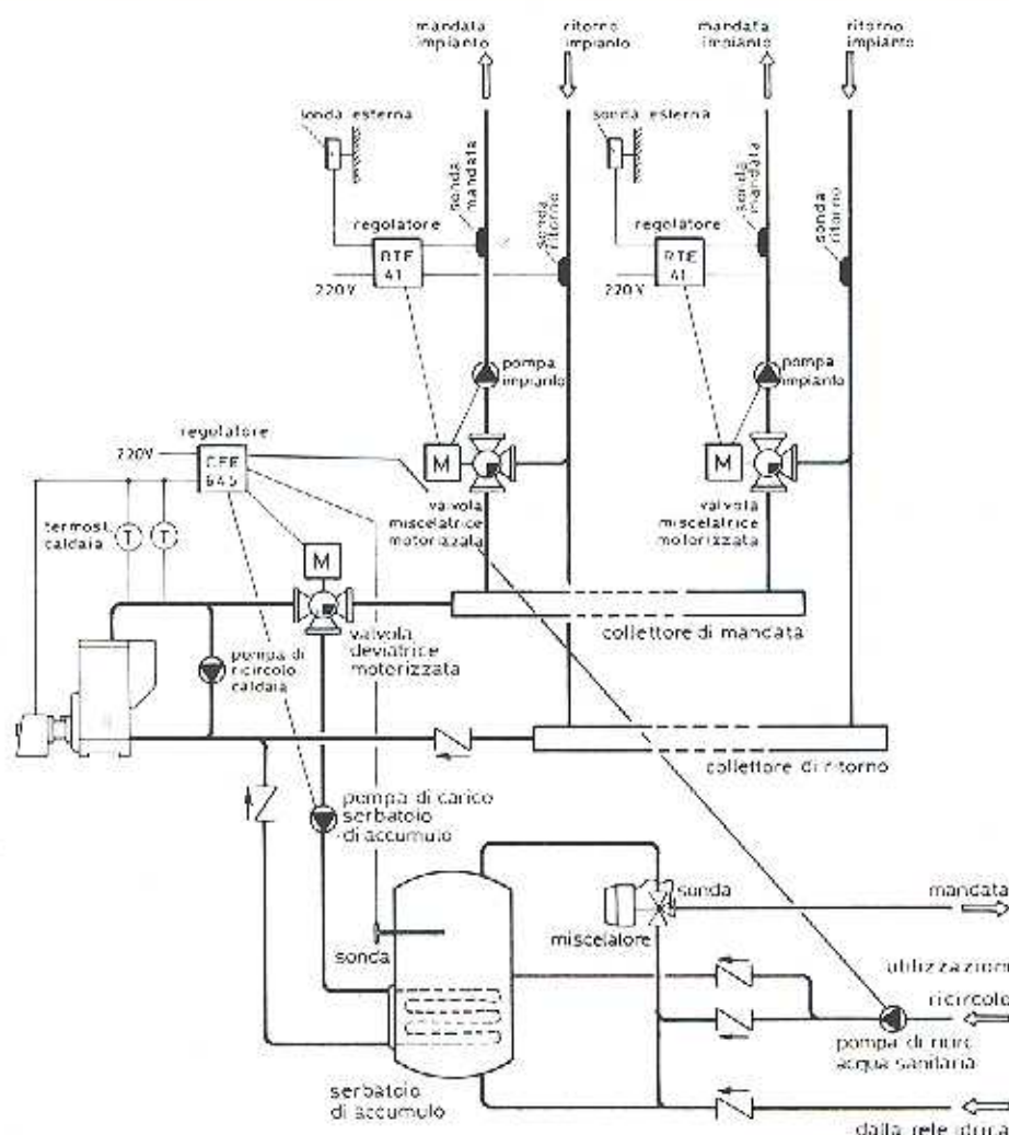
Impianto termico con produzione di acqua calda.
